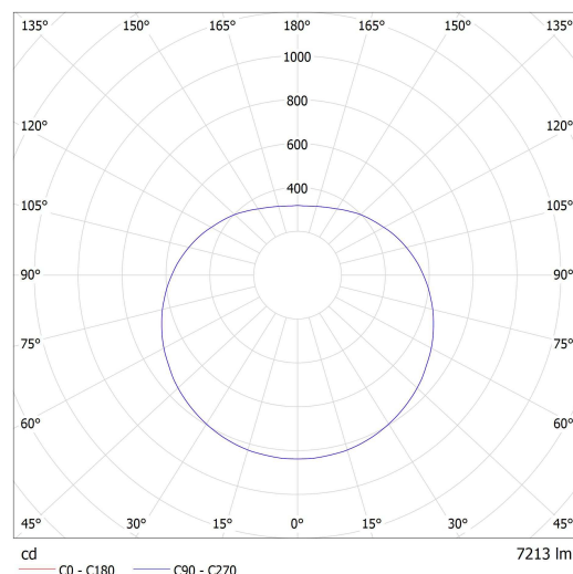
Lucis ZT.P2.630.X PE POLARIS ZT PE LED / LDC (Polar)
