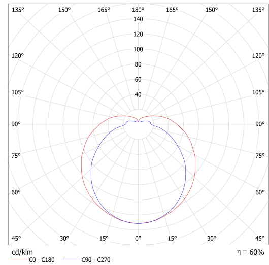
Lucis S1.12W PA MAIA / LDC (Polar)
