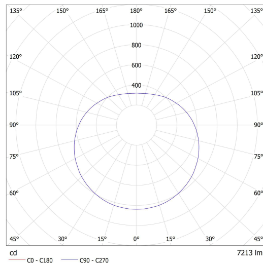
Lucis ZL1.P2.630.X PE POLARIS ZL PE LED / LDC (Polar)
