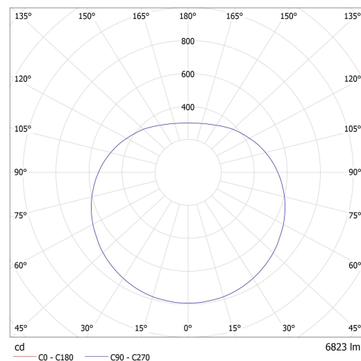
Lucis ZL1.P1.630.X PE POLARIS ZL PE LED / LDC (Polar)
