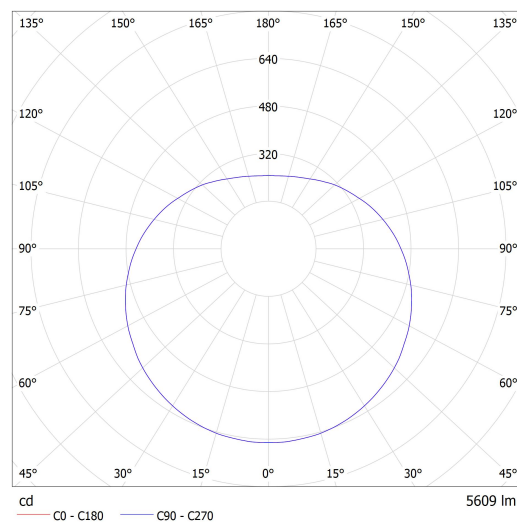
Lucis ZL1.P2.500.X PE POLARIS ZL PE LED / LDC (Polar)
