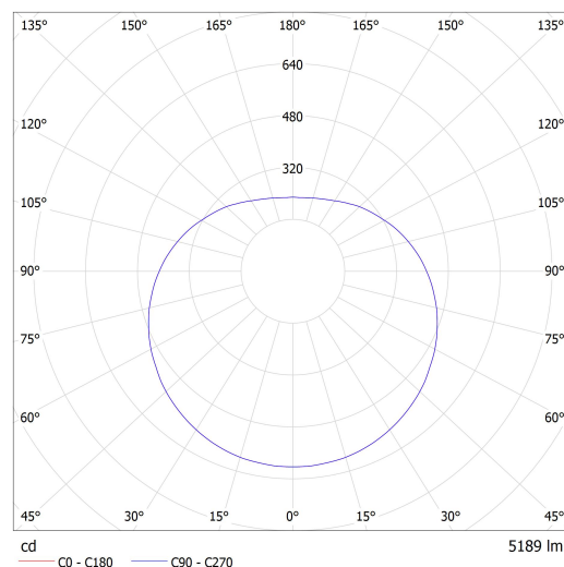
Lucis ZL1.P1.500.X PE POLARIS ZL PE LED / LDC (Polar)
