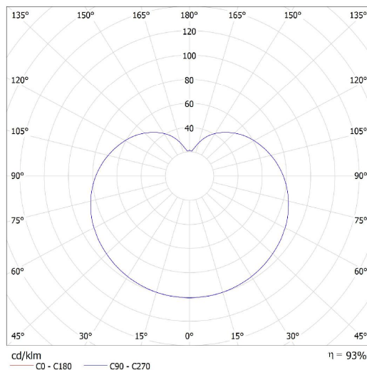
Lucis ZL1.11.500.X PE POLARIS ZL PE / LDC (Polar)
