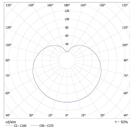
Lucis ZL1.11.400.X PE POLARIS ZL PE / LDC (Polar)
