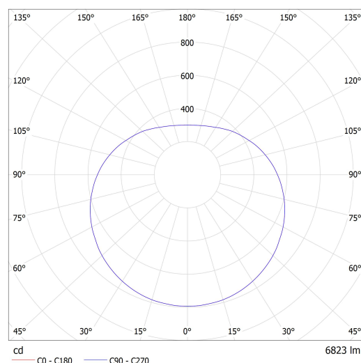
Lucis ZK.P1.600.X PE POLARIS ZK PE LED / LDC (Polar)
