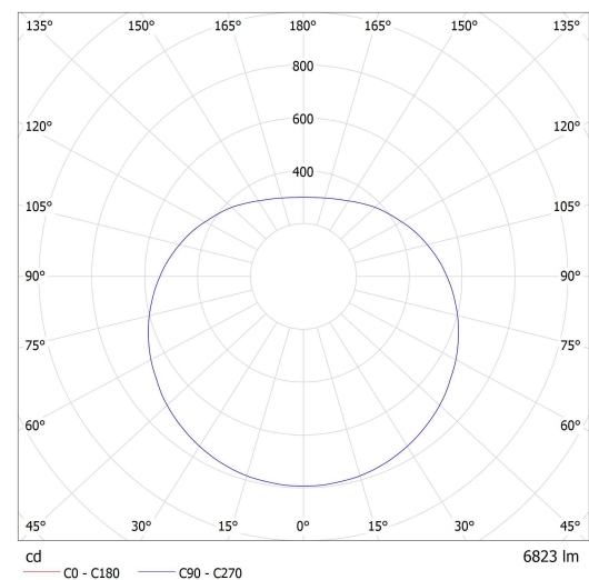
Lucis ZK.P1.630.X PE POLARIS ZK PE LED / LDC (Polar)
