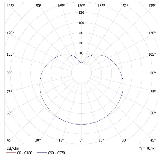
Lucis ZT.11.300.X PE POLARIS ZT PE / LDC (Polar)
