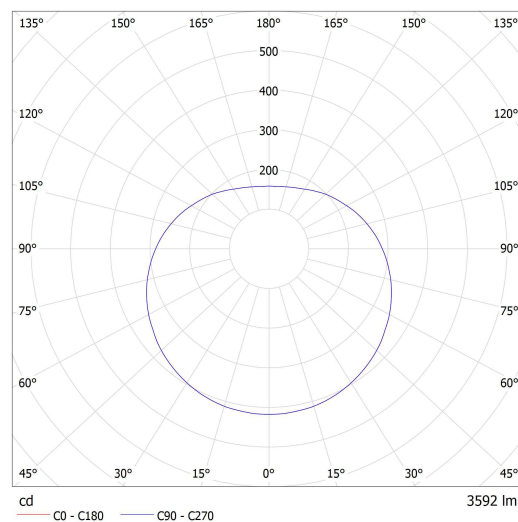
Lucis ZK.P1.400.X PE POLARIS ZK PE LED / LDC (Polar)
