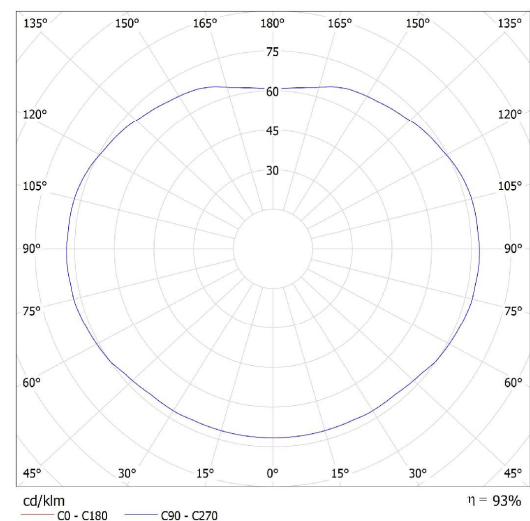
Lucis ZK.11.300.X POLARIS ZK / LDC (Polar)
