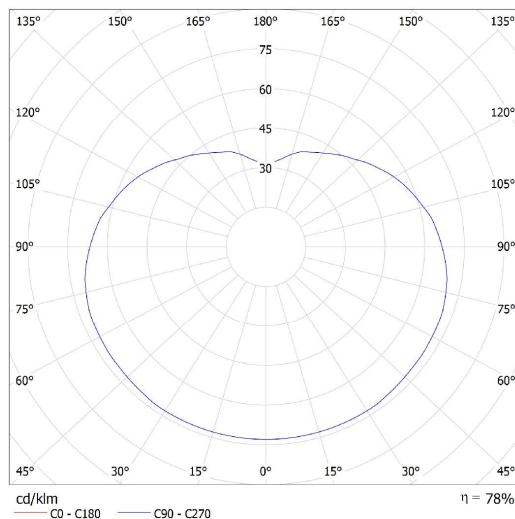
Lucis ZT.3X6.500 EVG POLARIS / LDC (Polar)
