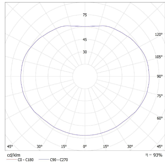
Lucis ZT.11.500.X POLARIS ZT / LDC (Polar)
