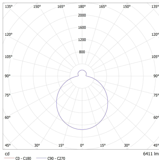
Lucis PS46.K2.O60 PE FORUM PE LED / LDC (Polar)
