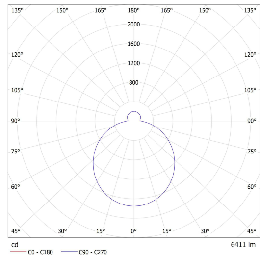
Lucis ZL3.K2.O60 PE FORUM PE LED / LDC (Polar)
