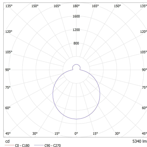
Lucis ZL3.K1.O50 PE FORUM PE LED / LDC (Polar)
