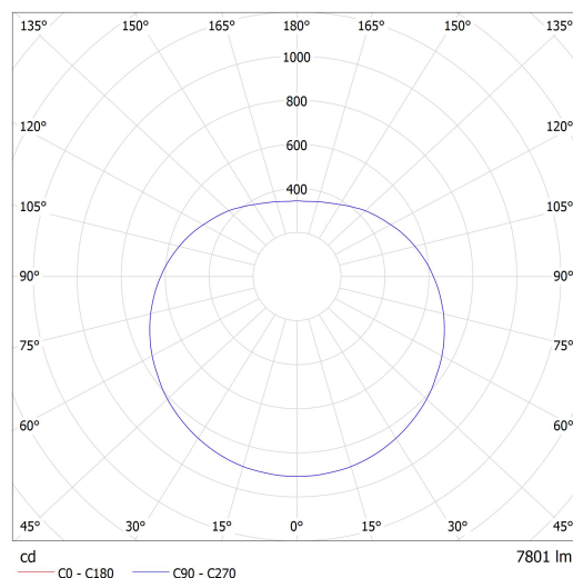
Lucis ZL1.P3.600.X PE POLARIS ZL PE LED / LDC (Polar)
