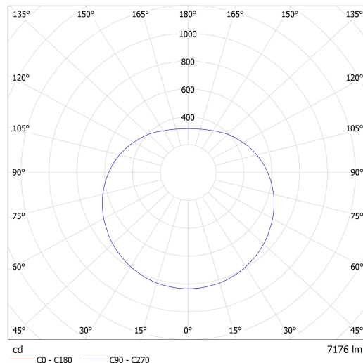
Lucis ZL1.P2.600.X PE POLARIS ZL PE LED / LDC (Polar)
