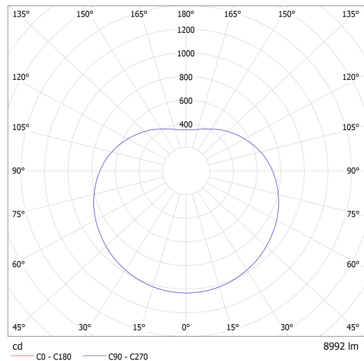
Lucis ZKS.P8.500.X POLARIS ZKS.P LED / LDC (Polar)
