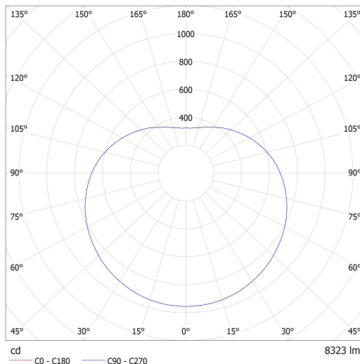
Lucis ZKS.P7.400.X POLARIS ZKS.P LED / LDC (Polar)
