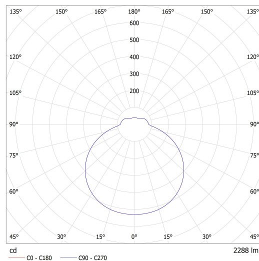
Lucis S33.K3.TEZ3 TENDO LED / LDC (Polar)
