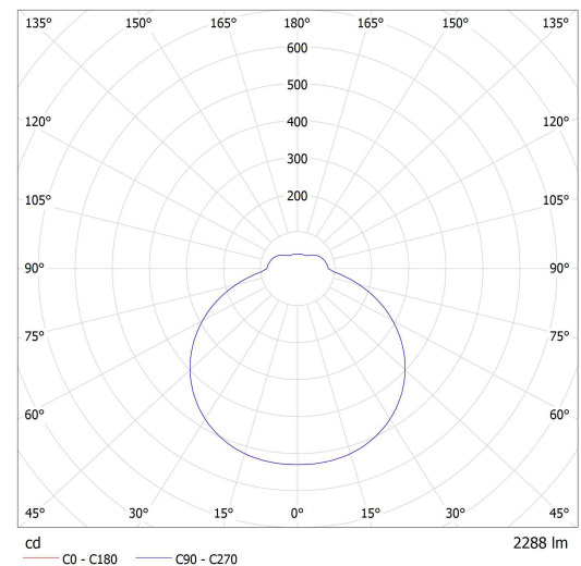
Lucis S33.K3.TEZ3 TENDO LED / LDC (Polar)
