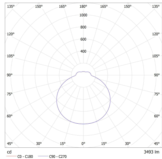
Lucis S33.K2.TEZ3 TENDO LED / LDC (Polar)
