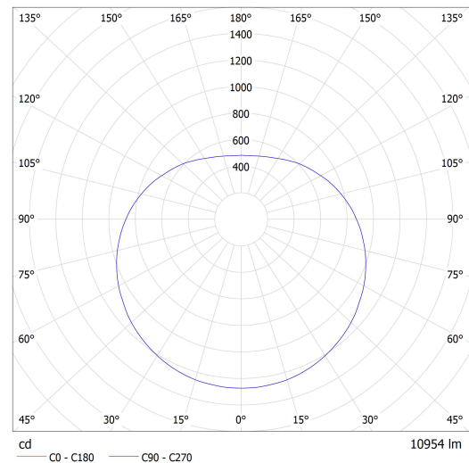
Lucis ZL1.P1.1000.X PE POLARIS ZL MAX PE LED / LDC (Polar)
