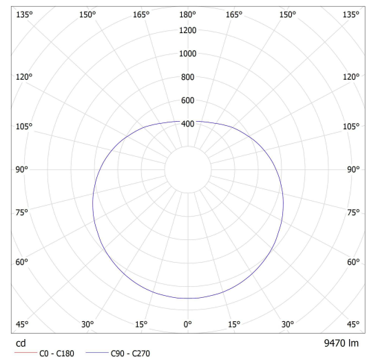
Lucis ZL1.P1.770.X PE POLARIS ZL MAX PE LED / LDC (Polar)
