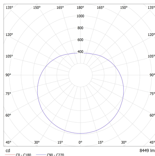
Lucis ZT.P3.630.X PE POLARIS ZT PE LED / LDC (Polar)
