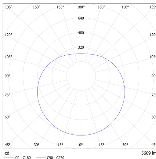
Luminaire: Lucis ZT.P4.400.X PE POLARIS ZT PE LED Lamps: 1 x LED G6
