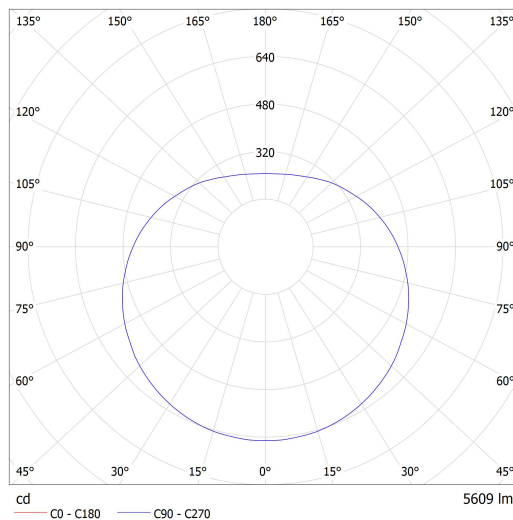
Lucis ZT.P4.400.X PE POLARIS ZT PE LED / LDC (Polar)
