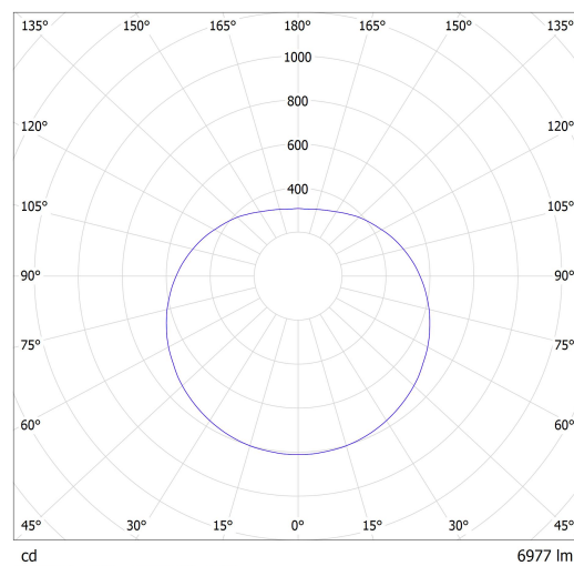
Lucis ZK.P3.600.X PE POLARIS ZK PE LED / LDC (Polar)
