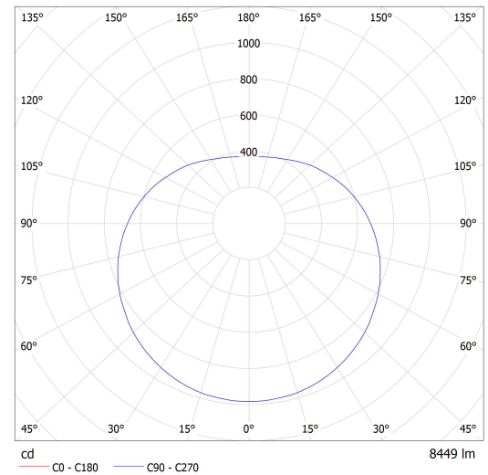
Lucis ZL1.P3.630.X PE POLARIS ZL PE LED / LDC (Polar)
